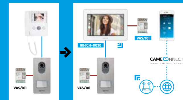
Alimentazione separata XTS e posto esterno
